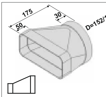
Uebergangstück 222x90 / D=150 Art.-Nr. 102.250.133 Fr. 49.40
