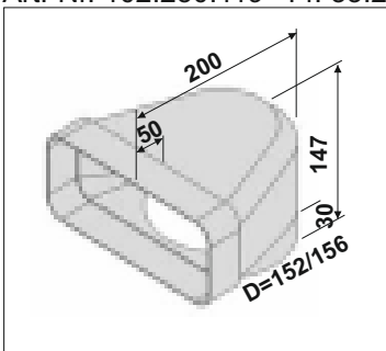
Umlenkstück 90° 222x90 / D=150 Art.-Nr. 102.250.129 Fr. 53.60
