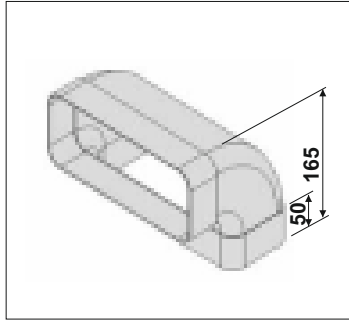
Bogen 90° vertikal 222x90 Art.-Nr. 102.250.131 Fr. 49.30
