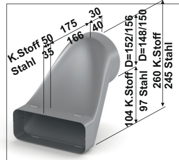
Versatzstück K.Stoff 222x90 / D=150 Art.-Nr. 102.252.136 Fr. 65.90 Versatzstück Stahl 222x90 / D=150 Art.-Nr. 102.252.135 Fr. 142.20
