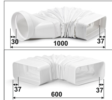
Bogen Flex 222x90 / D=150 Art.-Nr. 102.250.134 Fr. 71.60 Bogen Flex 222x90 / 222x90 Art.-Nr. 102.250.135 Fr. 68.80
