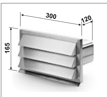
Wettergitter Inox mit Rückstauklappe 222x90 Art.-Nr. 102.252.141 Fr. 216.00
