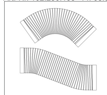
Flachkanal Alu/P Flex 222x90 0.5m Art.-Nr. 102.250.123 Fr. 24.00 1.0m Art.-Nr. 102.250.124 Fr. 48.00
